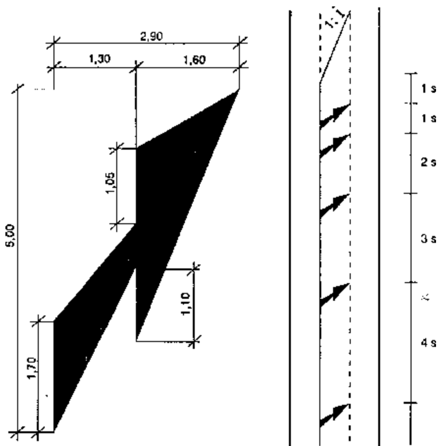
Размери на дясна стрелка
